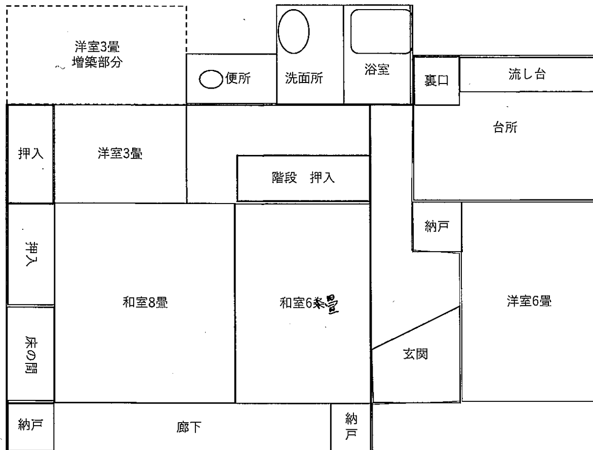
1 階 平面図
