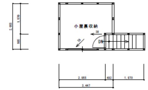
小屋裏収納平面図 S=1/100
