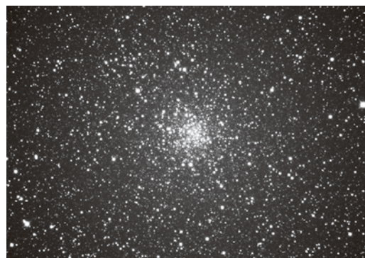
まんのう天文台で撮影した、や座の球状星団(M71)
