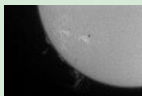
まんのう天文台で撮影した太陽
