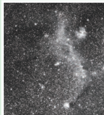
まんのう天文台で撮影したわし星雲
