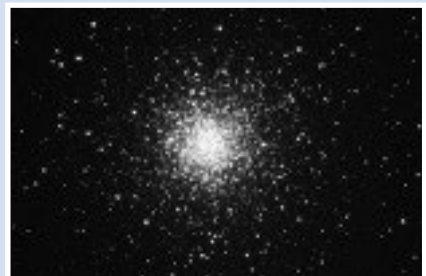
まんのう天文台で撮影した へびつかい座の球状星団
