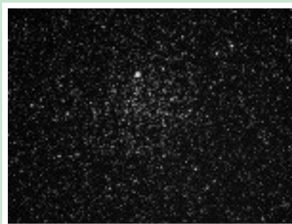
まんのう天文台で撮影した とも座の散開星団(M46)
