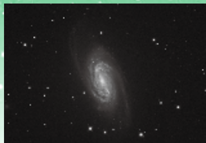
まんのう天文台で撮影した しし座の渦巻銀河(NGC2903)
