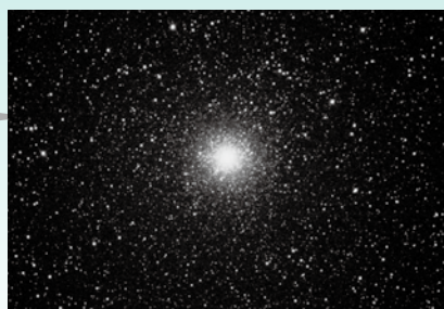
まんのう天文台で撮影した、いて座の球状星団(M54)
