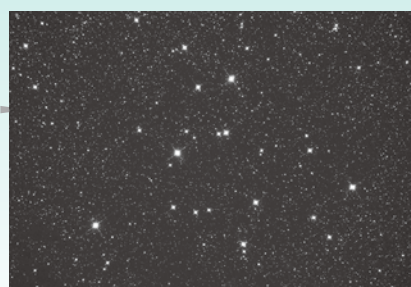
まんのう天文台で撮影した、はくちょう座の散開星団(M39)
