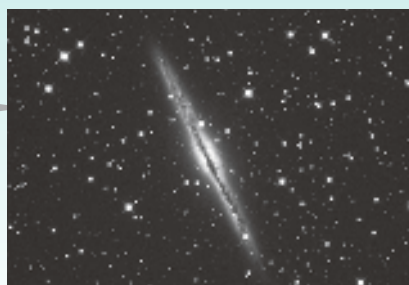
まんのう天文台で撮影した、アンドロメダ座の渦巻銀河(NGC891)
