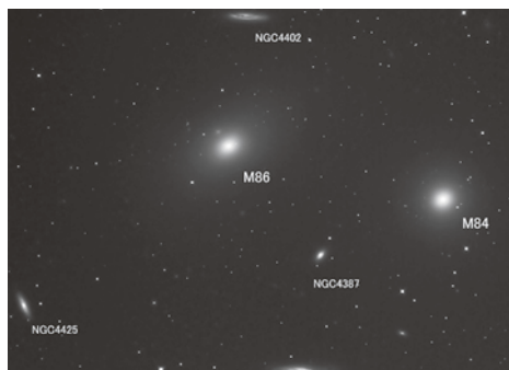
まんのう天文台で撮影した、マルカリアン銀河鎖(M84+86)
