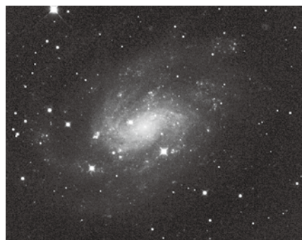
まんのう天文台で撮影した、ちょうこくしつ座の渦巻銀河(NGC300)
